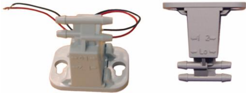
Autozero Module.
